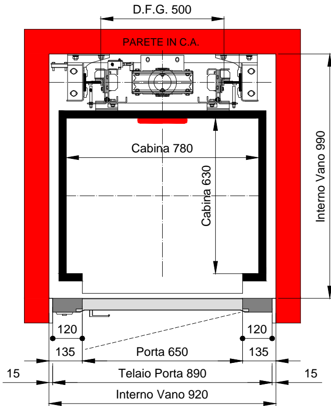
PIANTA VANO CORSA
